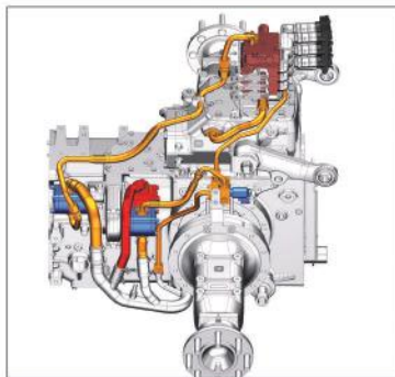
NA ZAHTEV 90 l/min HIDRAULIČKI SISTEM
