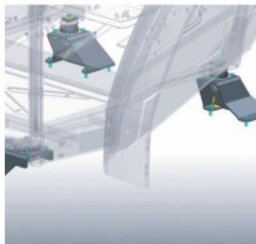
HIDRO SILENT BLOK SUSPENZIJA KABINE
